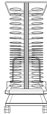
QUICK.PLATE para hornos 20 GN 2/1 - 102 platos 776 x 851 x 1709 mm - l x a x a Art. XEVTL-102P para hornos 20 GN 1/1 - 51 platos 776 x 681 x 1709 mm - l x a x a Art. XEVTL-051P
